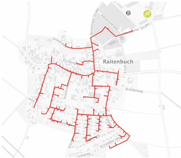
Abbildung 6: Bestandswärmenetz Raitenbuch (Veröffentlichung nach WPG, Anlage 2, I.)
